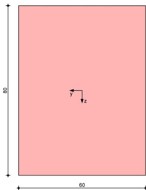
Querschnittsgrafik [cm]
